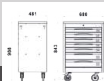
DIMENSIONI CASSETTO FG 102
